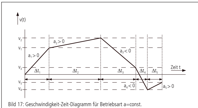
Bild 17: Geschwindigkeit-Zeit-Diagramm für Betriebsart a=\text{const.}
