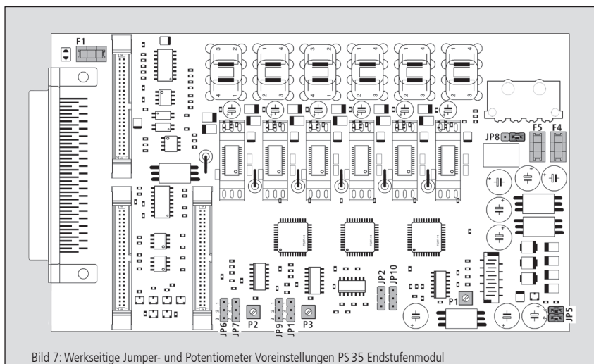
Bild 7: Werkseitige Jumper- und Potentiometer Voreinstellungen PS 35 Endstufenmodul
