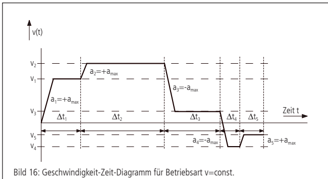
Bild 16: Geschwindigkeit-Zeit-Diagramm für Betriebsart v=\text{const.}
