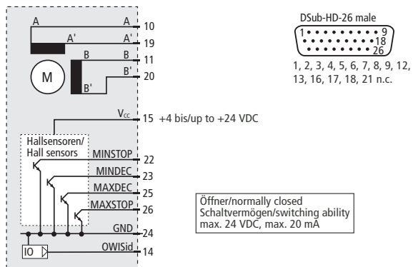
Steckerbelegung/pin configuration LIMES 170-XXXX-HiSM
