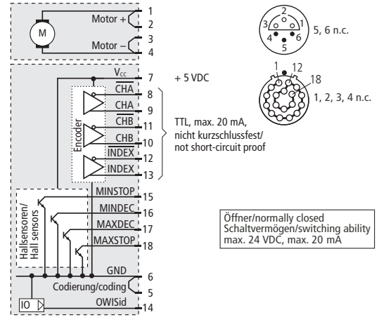
Steckerbelegung/pin configuration LIMES 170-XXXX-HiDS
